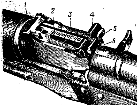
Рис. 28. Прицел:
