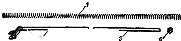
Рис. 33. Возвратный механизм:
