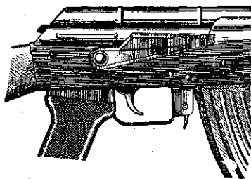
Рис. 53. Автомат поставлен на предохранитель
