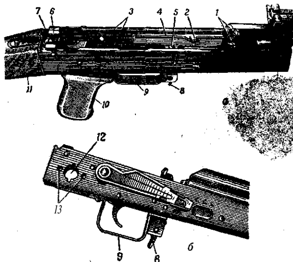
Рис. 27. Ствольная коробка:
