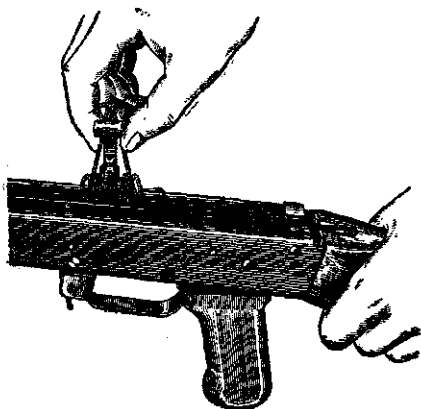
Рис. 17. Извлечение курка из ствольной коробки
