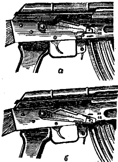
Рис. 58. Установка переводчика на необходимый вид огня: a — для ведения автоматического огня; б — для ведения одиночного огня
