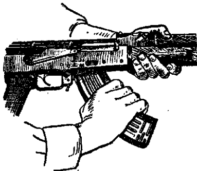
Рис. 11. Присоединение магазина
