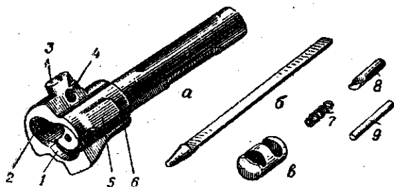
Рис. 32. Затвор:
