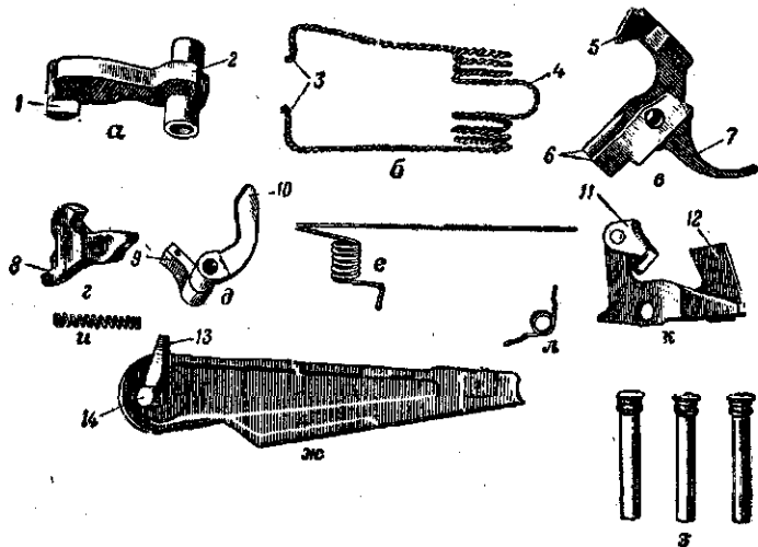
Рис. 35. Части ударно-спускового механизма:
