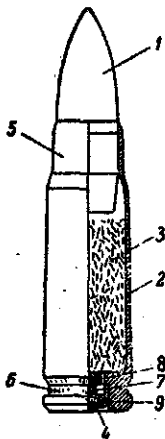
Рис. 41. Боевой патрон:
