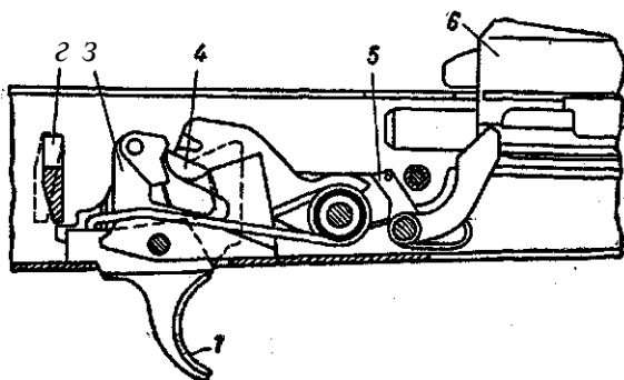
Рис. 44. Положение частей ударно-спускового механизма перед выстрелом:
