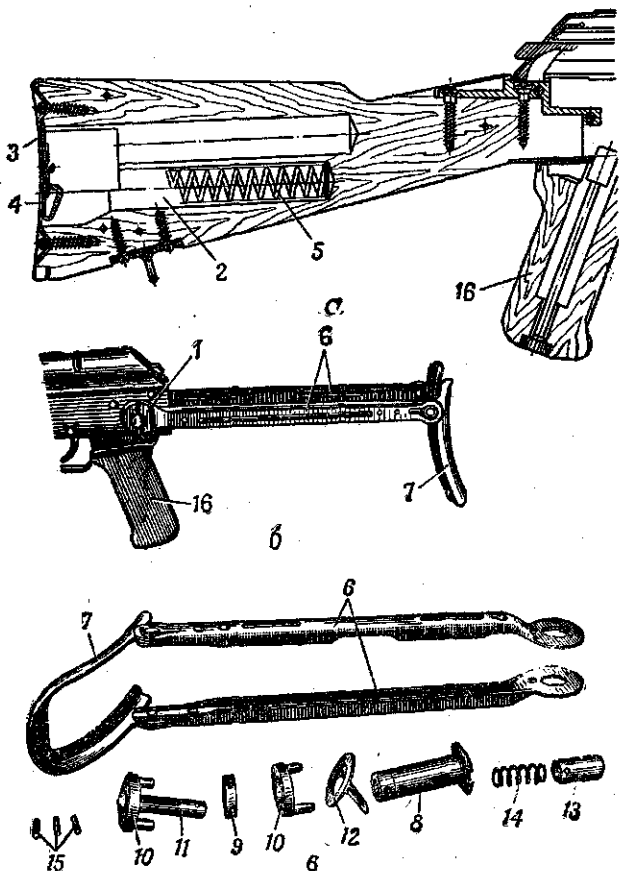
Рис. 30. Приклад и пистолетная рукоятка: a — деревянный приклад; б — складывающийся приклад: в — складывающийся приклад в разобранном виде; 1 — антабка для ремня; 2 — гнездо для принадлежности; 3 — затыльник; 4 — крышка; 5 — пружина для выталкивания пена-ла с принадлежностью; 6 — тяги; 7 — плечевой упор; 8 — соединительная втулка; 9 — гайка; 10 — фиксаторы приклада; 11 — соединительный стержень; 12 — шайба с антабкой; 13 — колпачок; 14 — пружина; 15 — шпильки; 16 — пистолетная рукоятка
