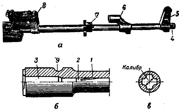
Рис. 25. Ствол:
