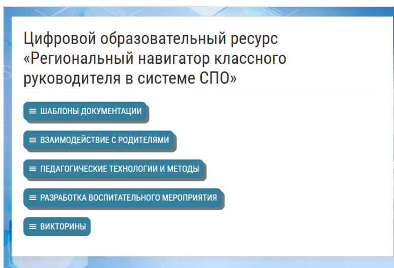
Рис.1 Интерфейс ЦОР
